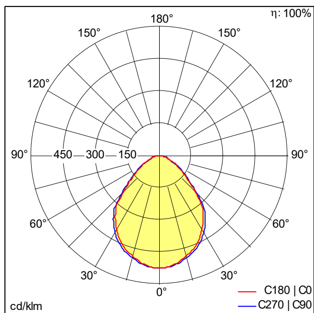
D33718_SLOT1_2_SLOT1_B_830_L1500_LRO_LDE.Idt
