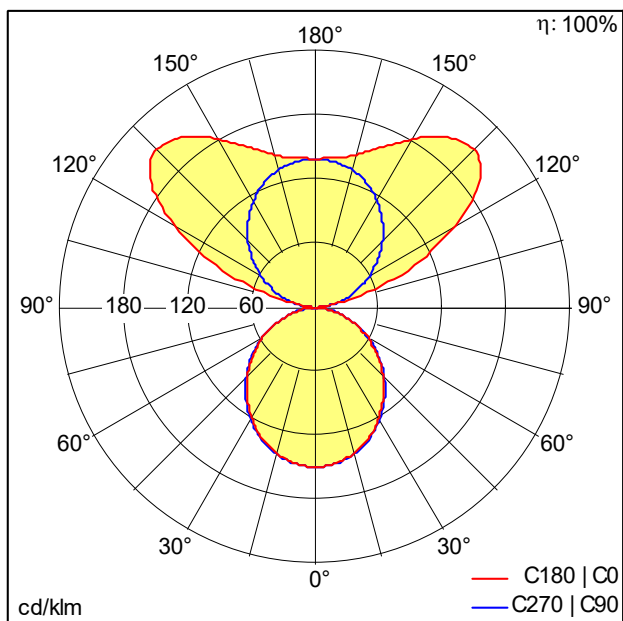
D42843AA_D44967AA_SLOIN_SLIM_ID_830_L2500_PC_WH.Idt
