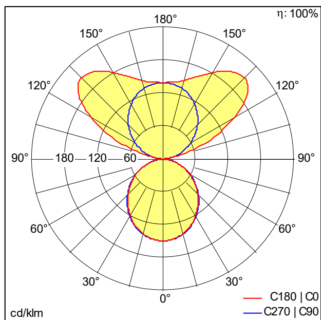
D42843AA_D44967AA_SLOIN_SLIM_ID_827_L2000_PC_WH.Idt
