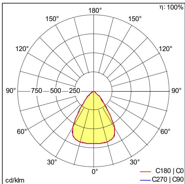
D49209_SLN2-B_2500-Z40_L1250_MC_LDE_SRM.Idt
