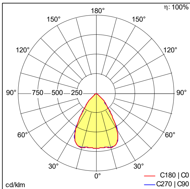
D49205_SLN2-B_2500-Z40_L1750_MC_LDE_SRG.Idt
