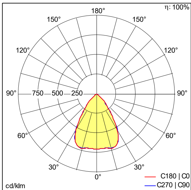
D49205_SLN2-B_2500-Z40_L2000_MC_LDE_SRG.Idt
