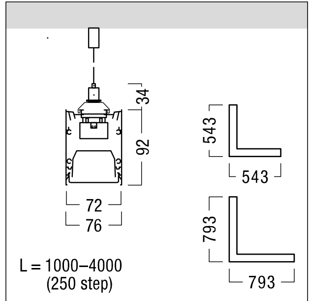
ZS_SL2_M_MSP_Corner.wmf
