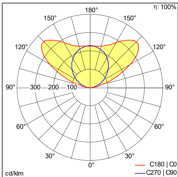
D46413_SLN2-C_2500-ZTW_L2000_BK_WW.Idt
