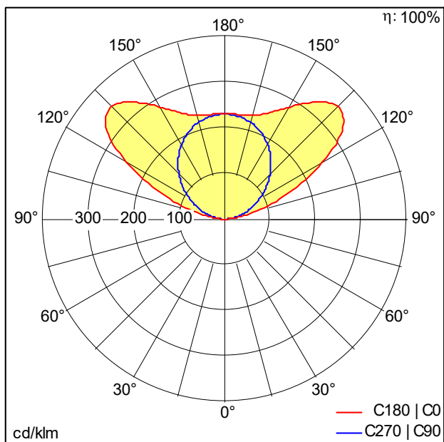
D46423_SLN2-C_2500-ZTW_L2000_WH_WW.Idt
