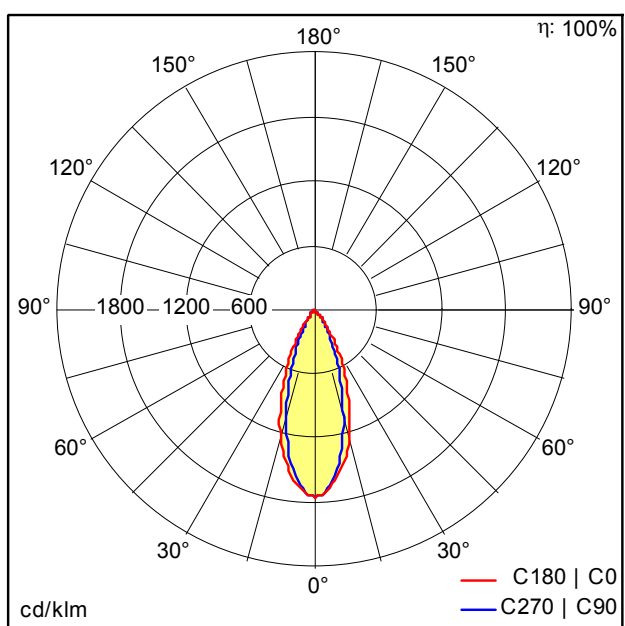
STx208.Idt
