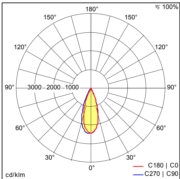
TE_LILY_LED_SPOT_IP44_38_68_600_927.ltd
