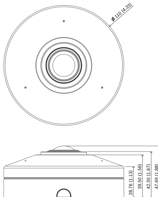
Dimensions en mm (pouces)
