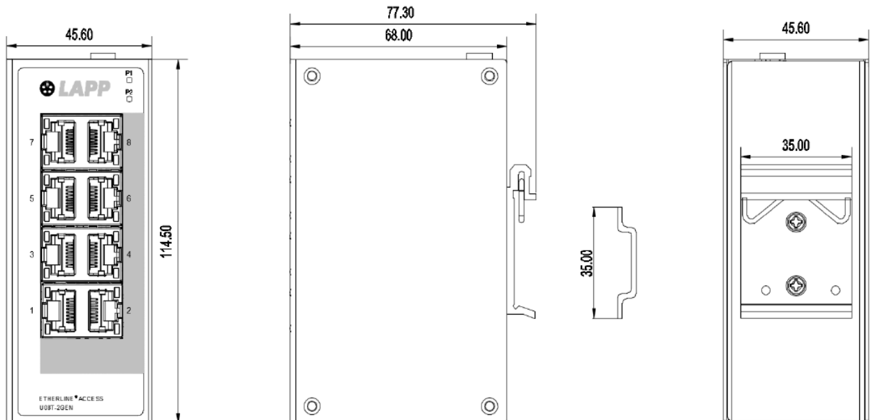
Maßzeichnung (U08T-2GEN)
