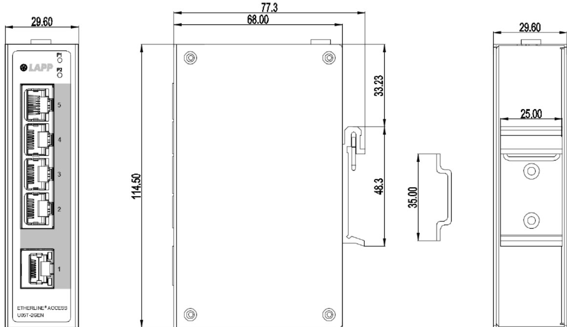
Maßzeichnung (U05T-2GEN)
