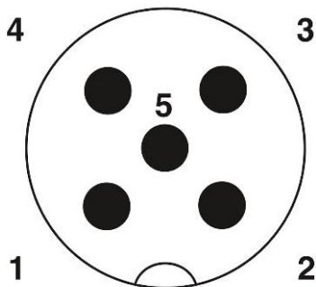
Pin assignment M12-plug, 5-pol, A-codiert
