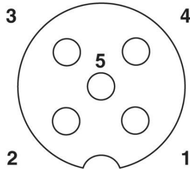
Pin assignment M12-jack, 5-pol, A-codiert
