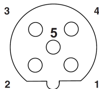
M12-Buchse, 5-polig, B-kodiert
