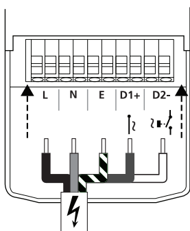
4a 220-240V~ + Switch-Dim
