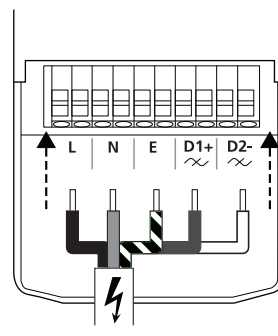
4c 220-240V~ + DALI
