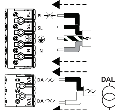
9d 220-240V~ + ⚡ + DALI ~
