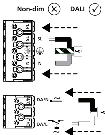
9e 220-240V~ + ~ Switch-Dim
