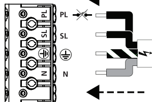
9b 220-240V~ + ⚡
