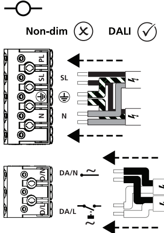
9f 220-240V~ + ~ Switch-Dim
