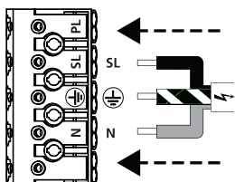
9a 220-240V~
