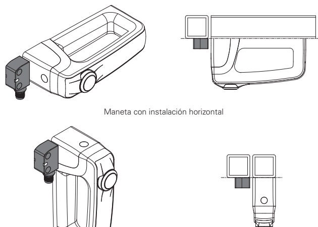
Maneta con instalación vertical
