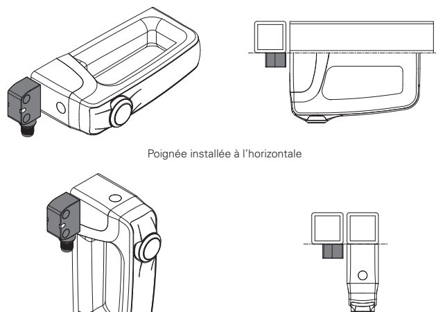
Poignée installée à la verticale
