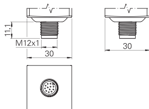
Connecteur M12 axial
