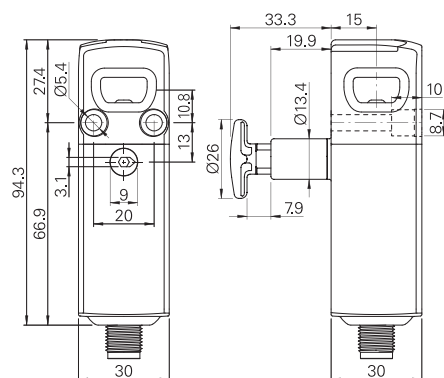
Dispositif NX ●●●AE●SMK
