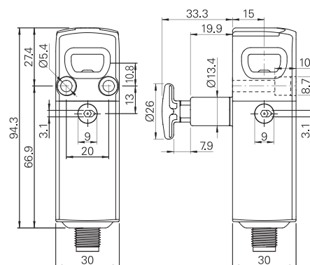
Dispositif NX ●●●CE●SMK
