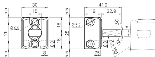
Actionneur VN NX-F●●
