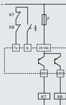
Zpětnovazební obvod pro externí stykače s ručním nebo monitorovaným startem
