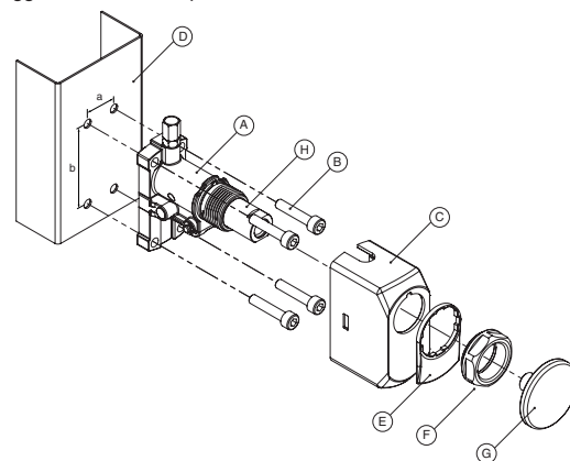
Fissaggio all'esterno del profilo
