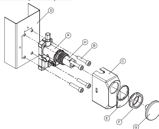
Montáž na vnější stranu profilu
