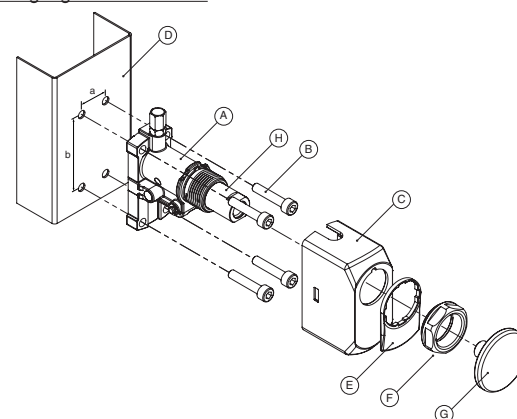
Befestigung außen am Profil
