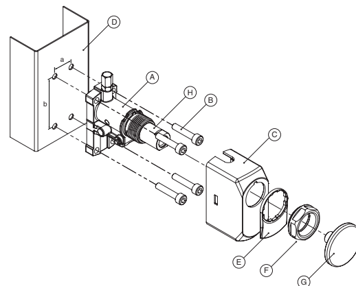
Fixation à l'extérieur du profil
