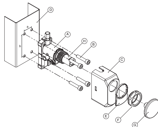
Fijación en el exterior del perfil
