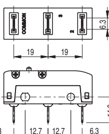
Bornes à cosses faston H verticales
