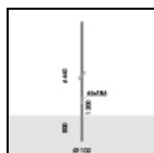
S.2815 POTEAU CYLINDRIQUE H 6,44m Ø102mm Poteau cylindrique comprenant : fût droit à section circulaire, diamètre 102 mm , épaisseur 4 mm, longueur totale 7,24 m , tronc unique construit en utilisant des tubes soudés à induction de façon longitudinale (ERW) UNI EN 10219-2-ISO 4200.
