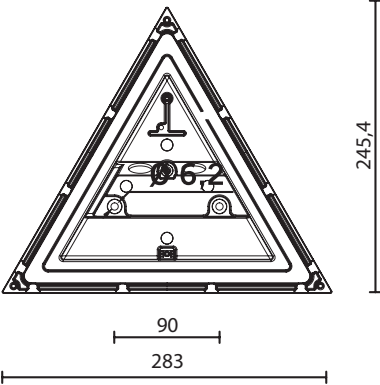
FIXING BASE BASE DI FISSAGGIO MONTAGEPLATTE BASE DE FIXATION
