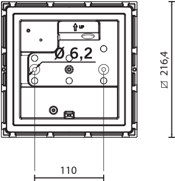
FIXING BASE BASE DI FISSAGGIO MONTAGEPLATTE BASE DE FIXATION
