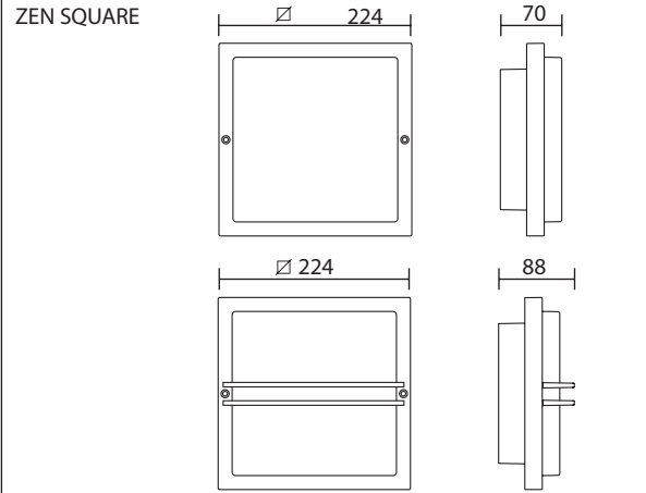
FIXING BASE BASE DI FISSAGGIO MONTAGEPLATTE BASE DE FIXATION
