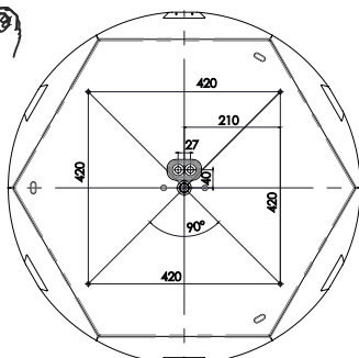
Bohrbild Hole pattern Trous de fixation Schema di foratura
