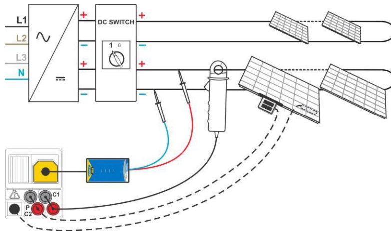
Schéma 6.15 : Test du panneau PV
