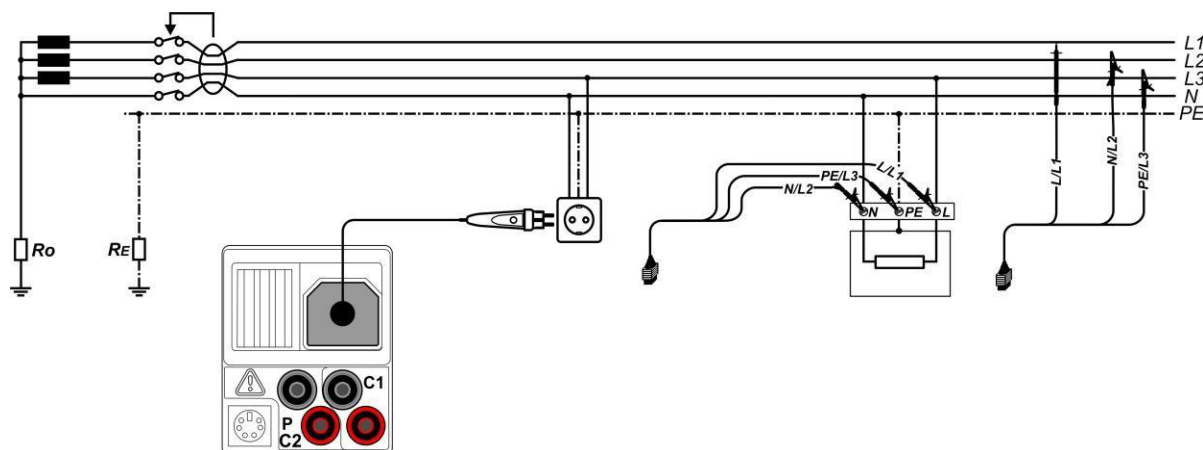
Schéma 5.3 : Connexion de la sonde déportée type prise et du cordon universel sur un réseau monophasé
