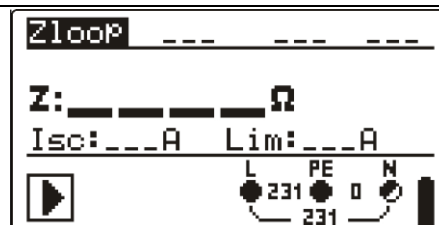
Schéma 5.23 : Impédance de boucle de défaut
