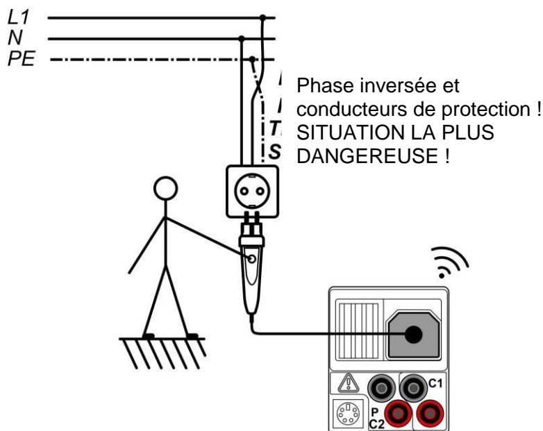
Schéma 5.36 : Conducteurs L et PE inversés (sonde active déportée)
