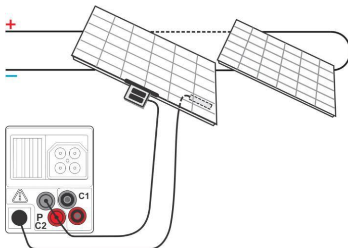
Schéma 6.18 : Mesure des paramètres environnementaux
