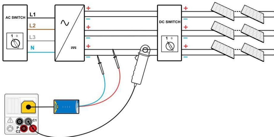
Schéma 6.6 : Test d'onduleur PV - côté DC
