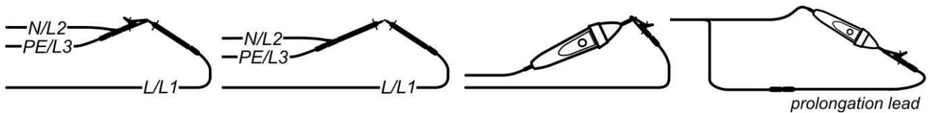
Schéma 5.13 : Court-circuiter les cordons de test
