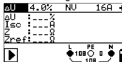
Schéma 5.27 : Chute de tension
