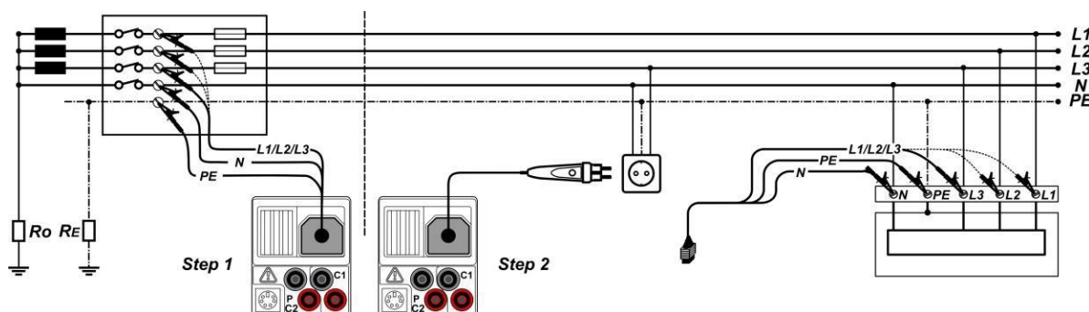
Schéma 5.30 : Mesure de l'impédance de ligne entre phase et neutre ou entre phase et phase – connexion de la sonde active 2P+T ou du cordon de test universel
