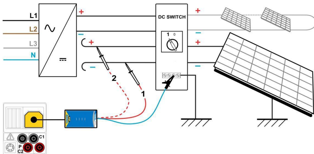
Schéma 6.2 : Paramètres de test pour la mesure de résistance d'isolement sur les systèmes PV
