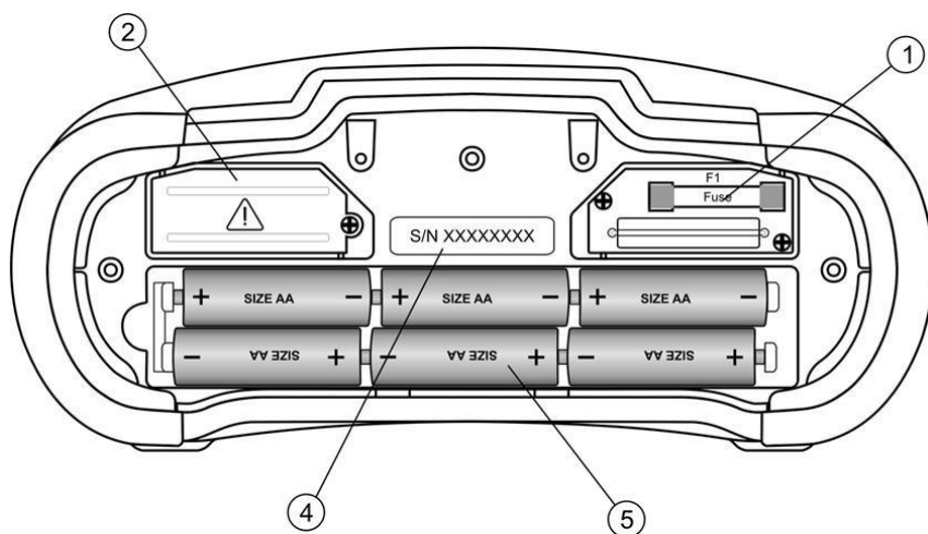
Schéma 3.4 : Compartiment piles et fusibles
