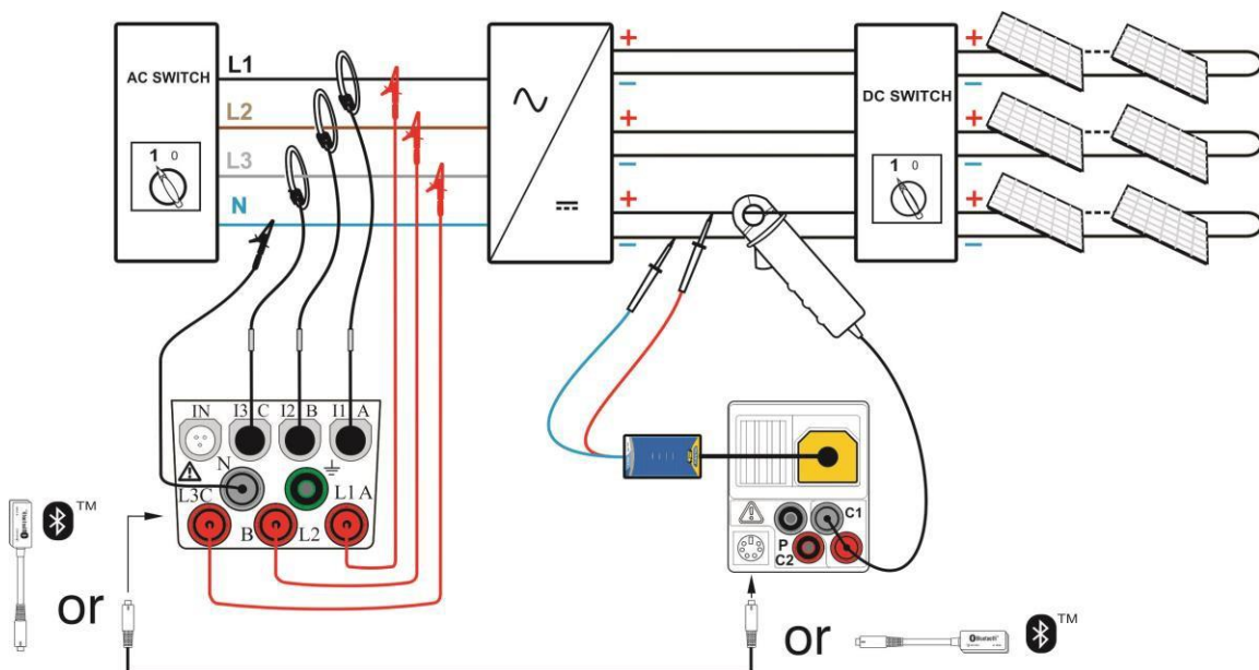
Schéma 6.10 : Test d'onduleur PV- triphasé côtés AC et DC
