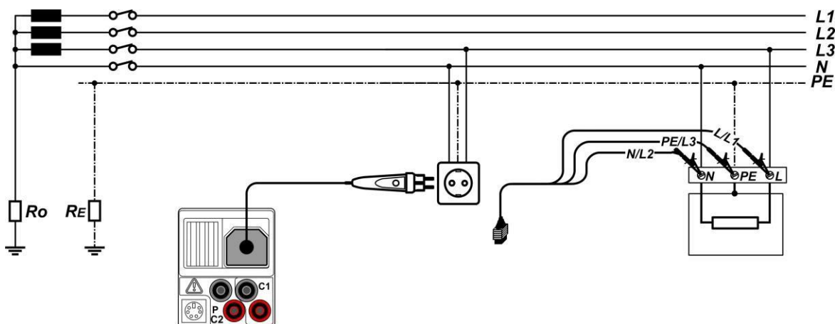
Schéma 5.24 : Connexion de la sonde active 2P+T ou du cordon de test universel
