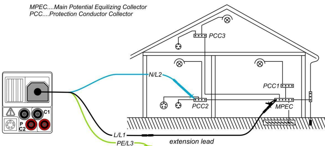
Schéma 5.9 : Connexion du cordon de test universel et du cordon d'extension optionnel
