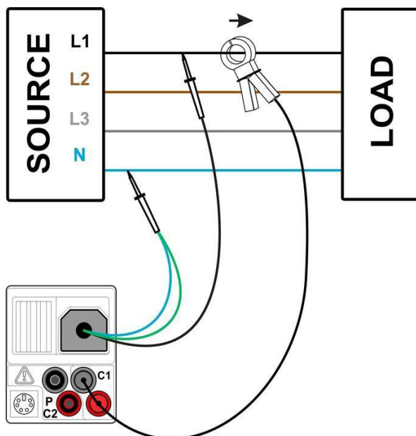
Schéma 7.2 : Mesure de puissance
