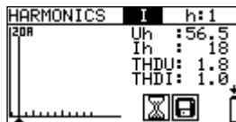
Schéma 7.5 : Exemples de résultats de mesure harmoniques
