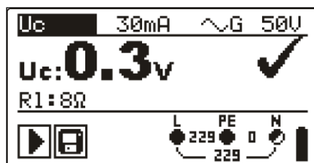
Schéma 5.18 : Exemple de résultats de mesure de tension de contact
