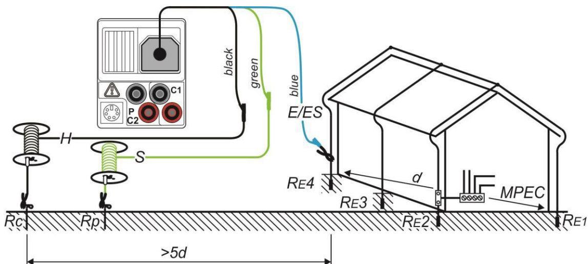
Schéma 5.34 : Résistance de terre, mesure de système de protection contre la foudre
