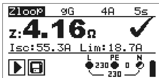
Schéma 5.25 : Exemple de résultat de mesure d'impédance de boucle
