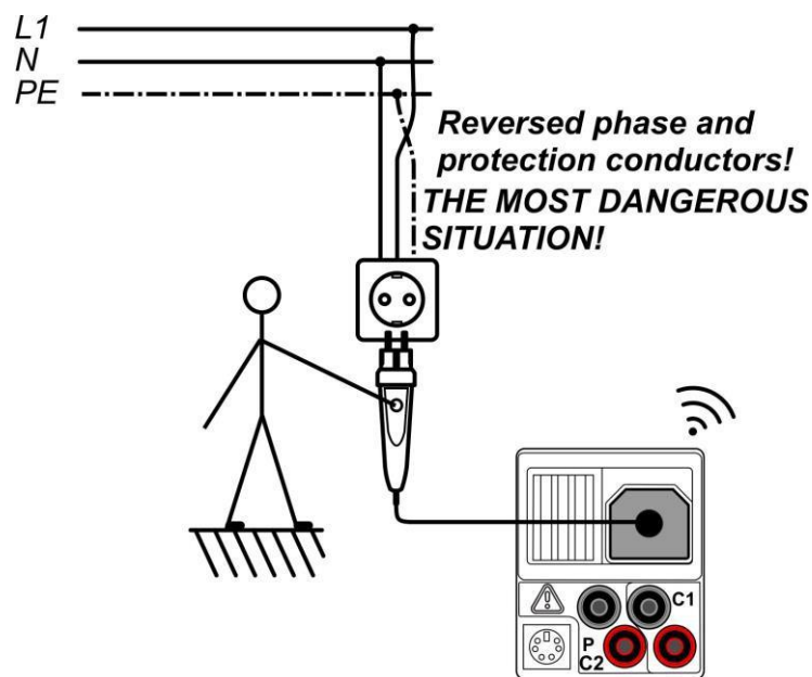
Schéma D.4 : Conducteurs L et PE inversés (application pour la sonde active 5P +T)
