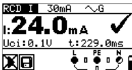
Schéma 5.20 : Exemples de résultats de mesure de courant de déclenchement,
