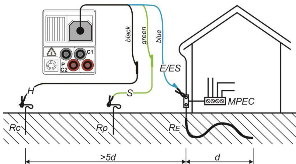
Schéma 5.33 : Résistance de terre, mesure de mise à la terre de l'installation principale
