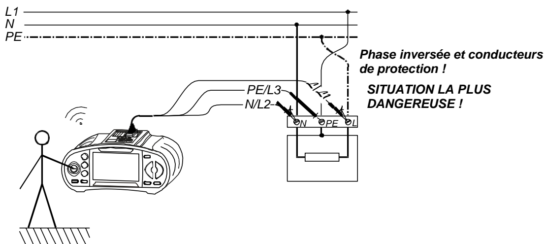
Schéma 5.37 : Conducteurs inversés L et PE (application avec le cordon de test universel)
