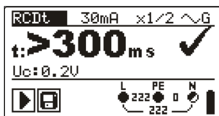
Schéma 5.19 : Exemple de résultats de mesure de déclenchement
