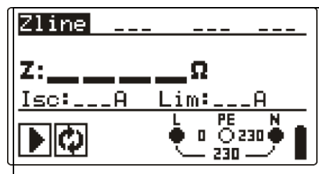
Schéma 5.26 : Impédance de ligne
