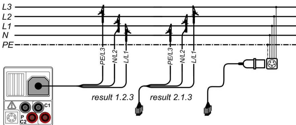
Schéma 5.2 : Connexion du cordon universel sur un réseau triphasé et de l'adaptateur triphasé optionnel
