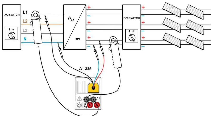
Schéma 6.8 : Test d'onduleur PV - côtés AC et DC
