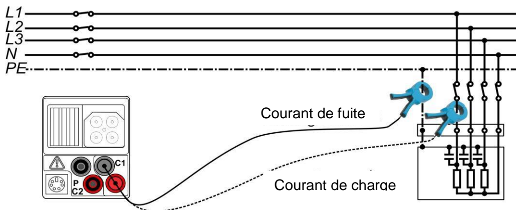
Schéma 7.9 : Mesures de courant de fuite et de courant charge,
