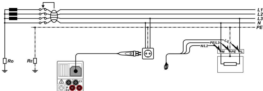
Schéma 5.17 : Connexion de la sonde déportée 2P+T ou du cordon de test universel
