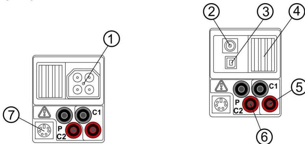
Schéma 3.2 : Bornier (image du MI 3108)
