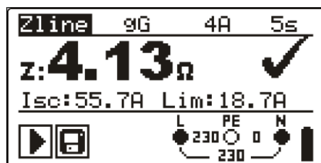
Schéma 5.29 : Exemple de résultat de mesure d'impédance de ligne
