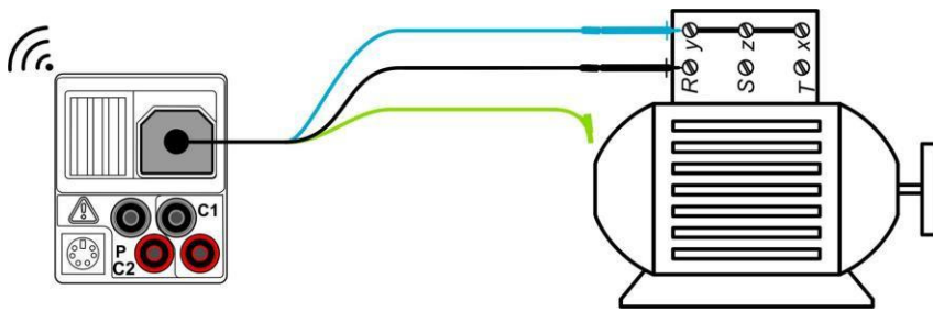
Schéma 5.11 : Connexion de la pointe de touche déportée optionnelle et du cordon de test universel
