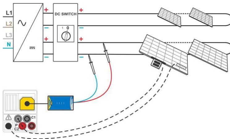
Schéma 6.22 : Test Uoc / Isc
