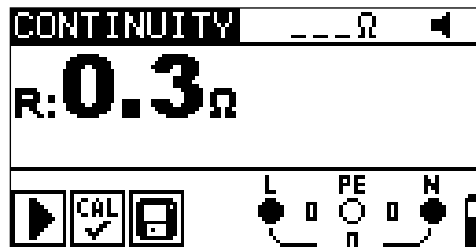
Schéma 5.12 : Exemple de mesure de résistance de continuité en continue
