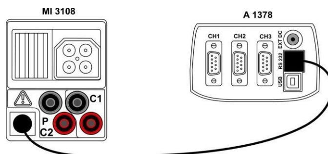
Schéma 4.19 : Connexion de l'appareil pendant la synchronisation
