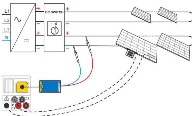
Schéma 6.25 : Teste de courbe I / V
