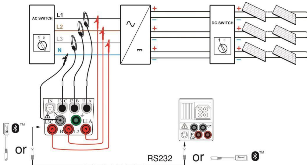
Schéma 6.9 : Test d'onduleur PV- triphasé - côté AC
