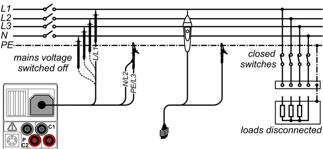
Schéma 5.6 : Connexions pour la mesure d'isolement
