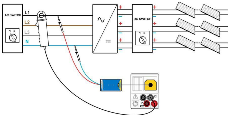
Schéma 6.7 : Test d'onduleur PV- côté AC
