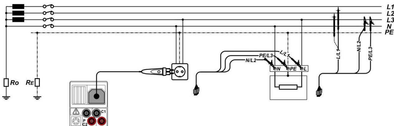
Schéma 5.28 : Mesure de l'impédance de ligne entre phase et neutre ou entre phase et phase – connexion de la sonde active 2P+T ou du cordon de test universel
