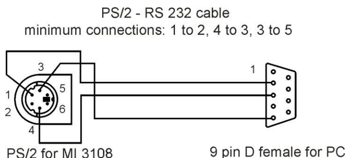
Schéma 8.14 : Connexion d'interface pour le transfert des données via le port COM du PC.
