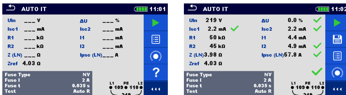
Image 4.117 : Exemples de résultats de mesure AUTO IT
