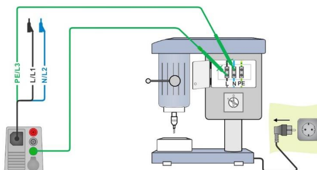
Image 4.104 : Mesure du temps de décharge
