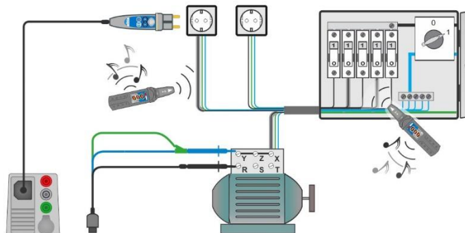
Image 4.119: Détections de câbles dans murs et armoires
