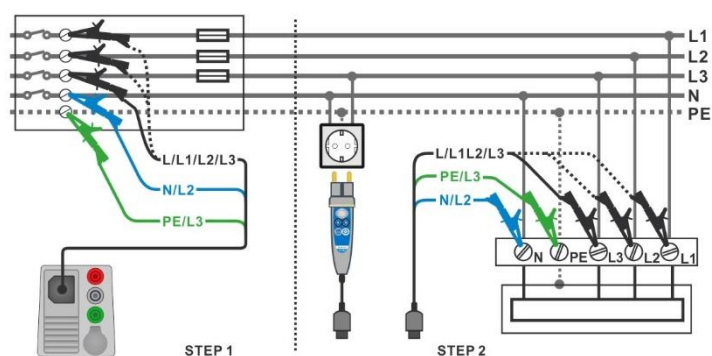
Image 4.107 : Mesure AUTO TT
