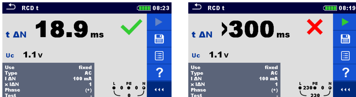
Image 4.36: Exemples de résultat de la mesure du temps d'ouverture
