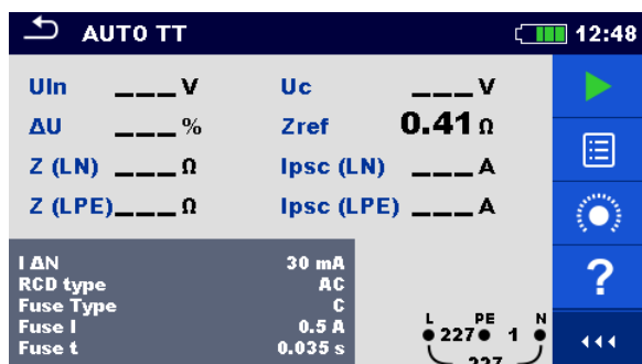
Image 4.108 : Exemples de résultats de mesure AUTO TT
