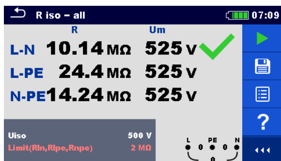
Image 4.12: Exemples de résultat de la mesure R iso - all
