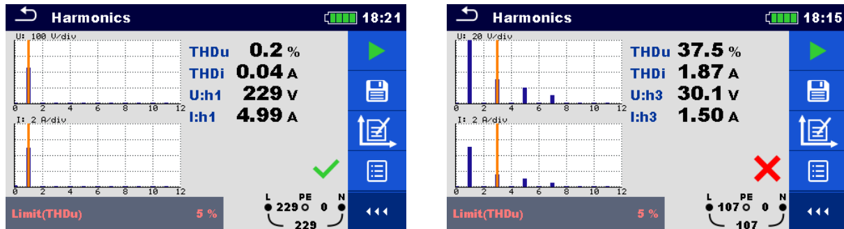
Image 4.85: Exemples de résultats de mesure d'harmoniques
