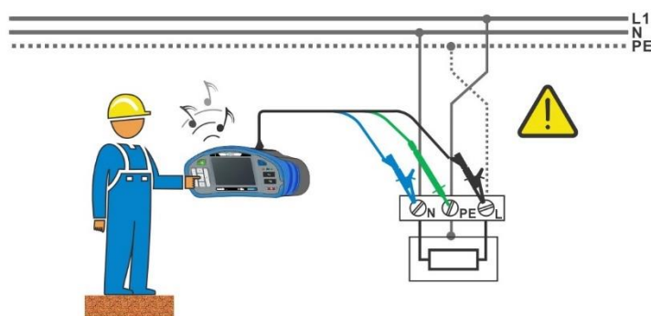
Image 1.2: Conducteur L et PE inversés (cordon de test 3 fils)
