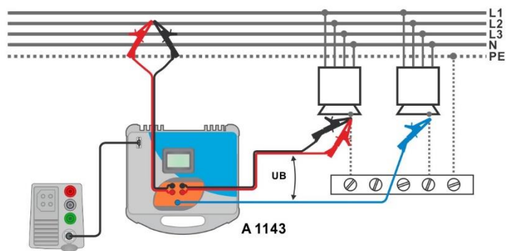
Image 4.52: Mesure Tension de contact– Connexion du A 1143
