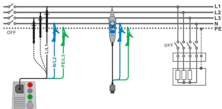
Image 4.11: Connection des cordons de test 3 fils avec Tip-commander
