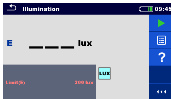
Image 4.99: Menu mesure d'éclairement
