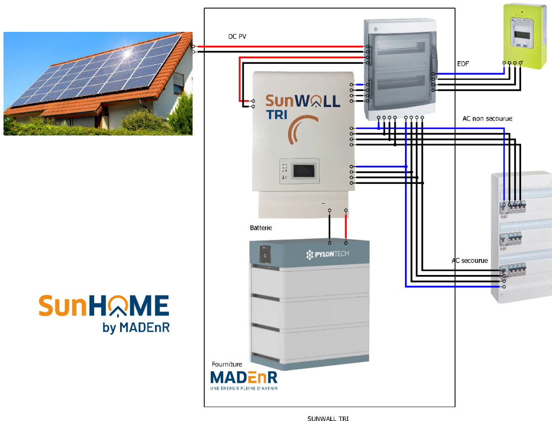
Figure 62 : Schéma de principe de la SunWall Tri
