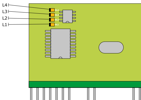
Figure 1 : Récepteur RF
