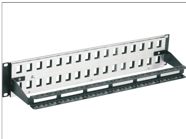
Panneau RJ45 VOL Everon® Datacom cuivre 19-pouce, 2 HE, flach, 32 Ports, schwarz
