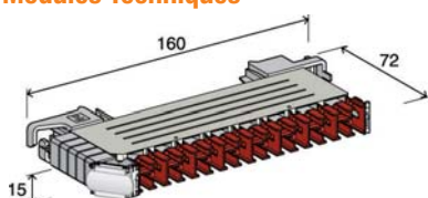
Module RIM
