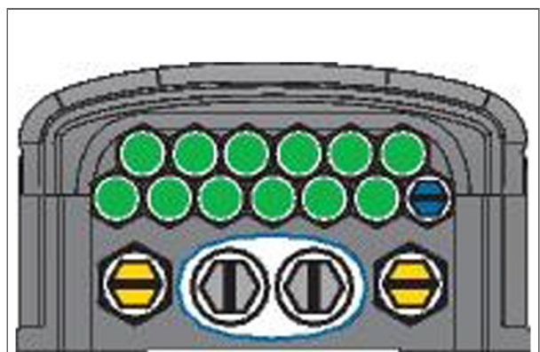
BPEO Boîtier de Protection d'épissures optiques, Taille 1.5 ECAM Connect 12 ports SC APC
