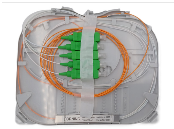
Cassette d'épissure K7, Cassette K7 1 Pas avec 1 Splitter 1x4 SC APC
