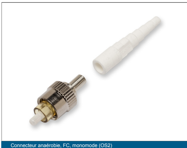
Connecteur anaérobie, FC, monomode (OS2)
