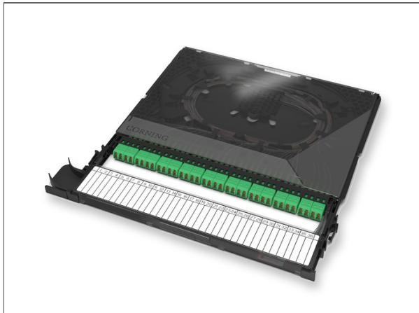
Cassette d'épissures Centrix®, 18 adaptateurs LC Duplex/APC et 36 pigtails LC/APC monofibre (OS2) HS
