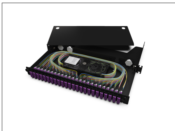
Tiroir optique Everon® LAN1, Face avant chargée avec épissures, LC Duplex, 96 Fibres, 1U, Multimode OM4, Casette d'épissures MFT pour sertir, protecteurs non inclus, noir
