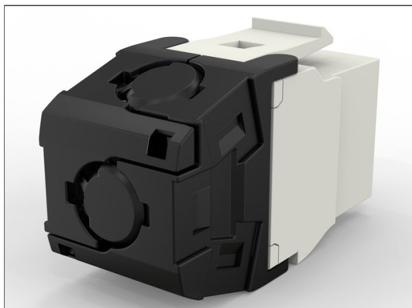
Connecteur non-blindé Everon® Datacom cuivre KS250S, Cat.6A, Keystone, pack de 6
