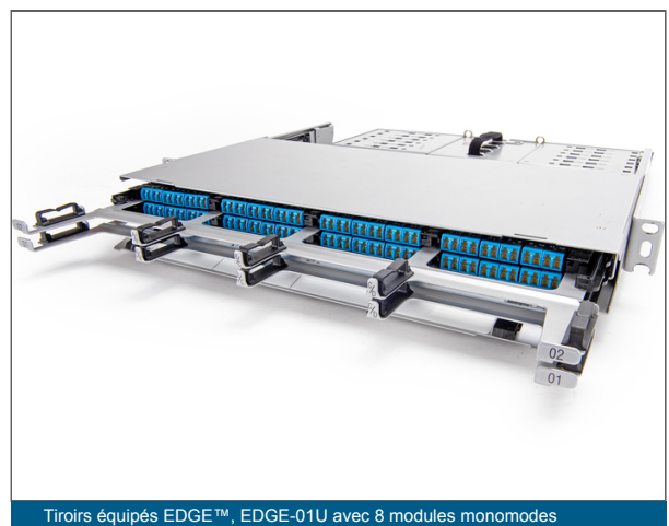
Tiroirs équipés EDGE™, EDGE-01U avec 8 modules monomodes
