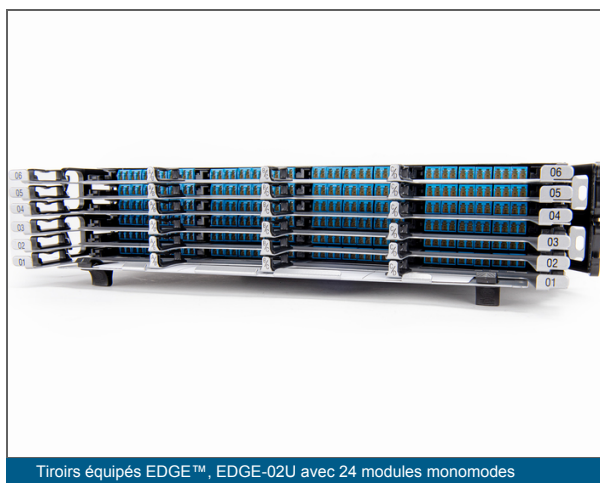
Tiroirs équipés EDGE™, EDGE-02U avec 24 modules monomodes
