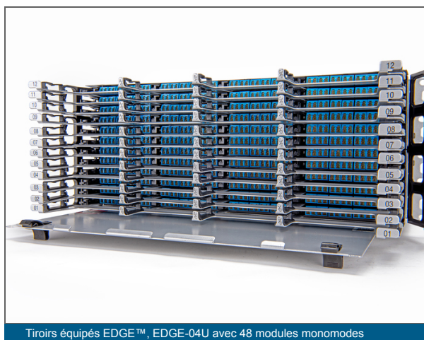
Tiroirs équipés EDGE™, EDGE-04U avec 48 modules monomodes
