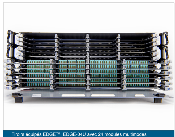
Tiroirs équipés EDGE™, EDGE-04U avec 24 modules multimodes
