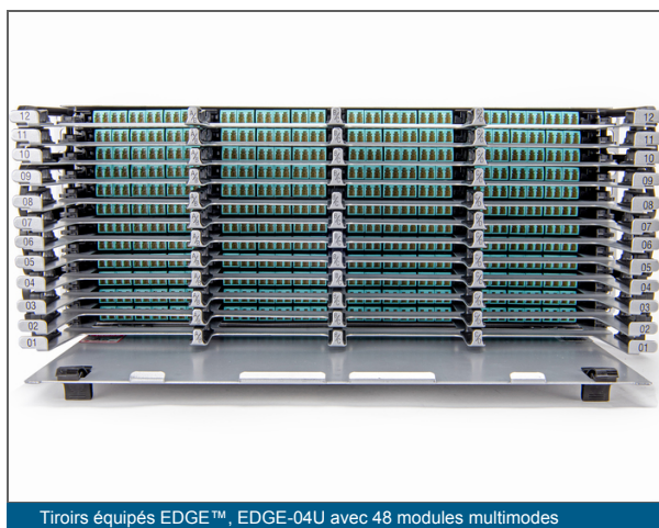
Tiroirs équipés EDGE™, EDGE-04U avec 48 modules multimodes
