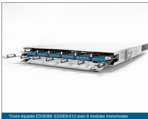
Tiroirs équipés EDGE8®, EDGE8-01U avec 6 modules monomodes
