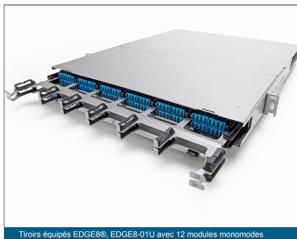
Tiroirs équipés EDGE8®, EDGE8-01U avec 12 modules monomodes
