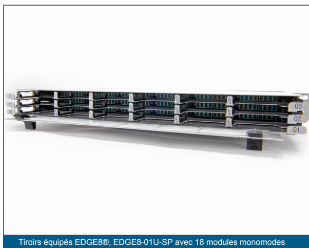
Tiroirs équipés EDGE8®, EDGE8-01U-SP avec 18 modules monomodes
