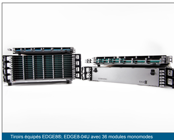
Tiroirs équipés EDGE8®, EDGE8-04U avec 36 modules monomodes
