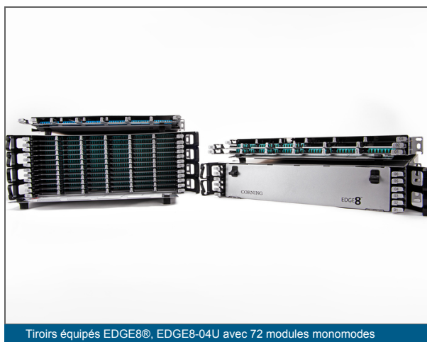
Tiroirs équipés EDGE8®, EDGE8-04U avec 72 modules monomodes
