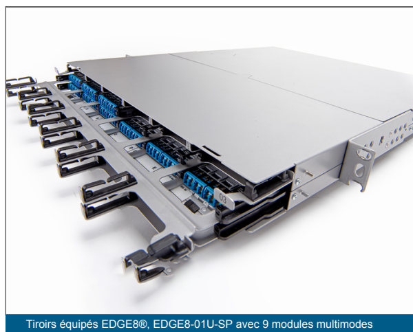
Tiroirs équipés EDGE8®, EDGE8-01U-SP avec 9 modules multimodes
