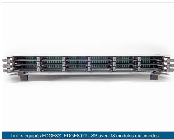
Tiroirs équipés EDGE8®, EDGE8-01U-SP avec 18 modules multimodes
