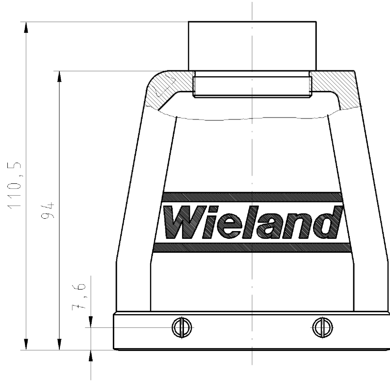
Ausführung .2 version .2
